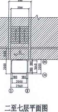
平面图2
