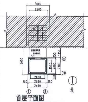
平面图1
