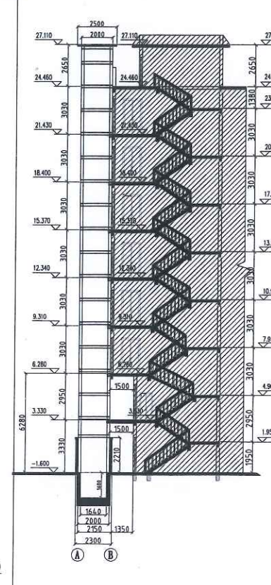
I-I剖面图
