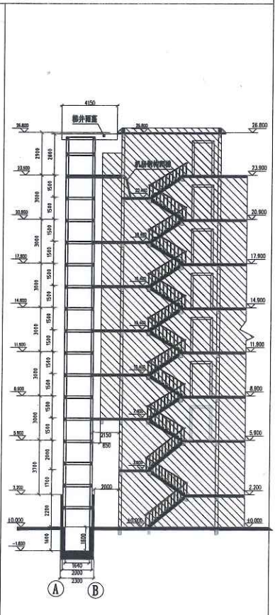
I-I剖面图
