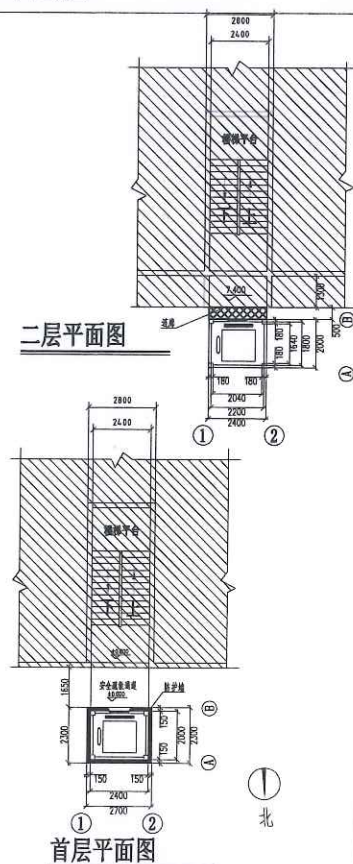
平面图1
