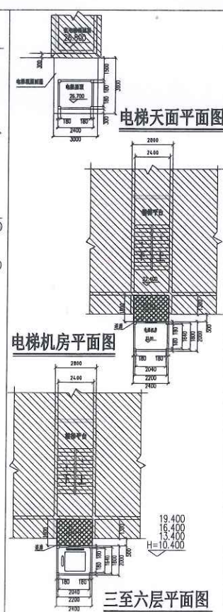
平面图2
