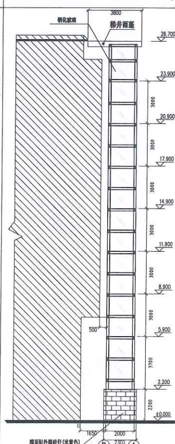
①-②轴立面图
