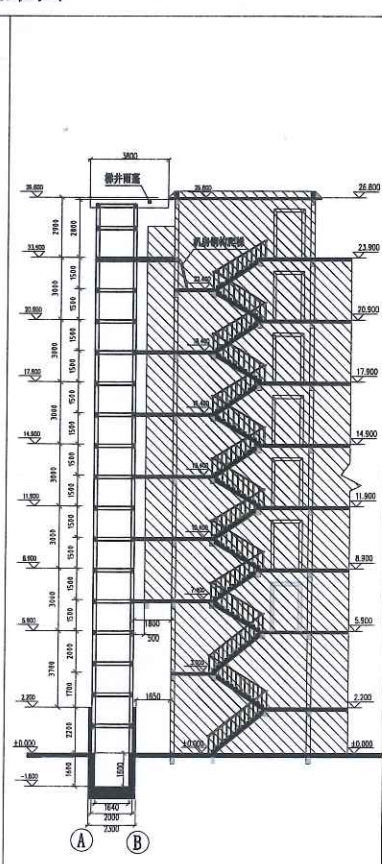
I-I剖面图
